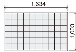
〈CS-320G31 外形図〉
