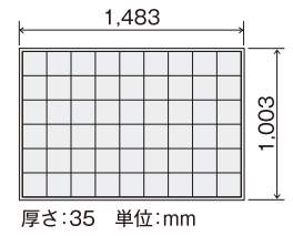
〈CS-282G31 外形図〉
